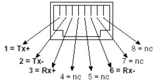
Abb. 8: RJ45-Buchse (Belegung AT&T256)
